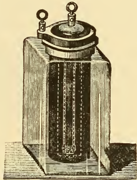
FIG. 101. — Léclanche cell.
